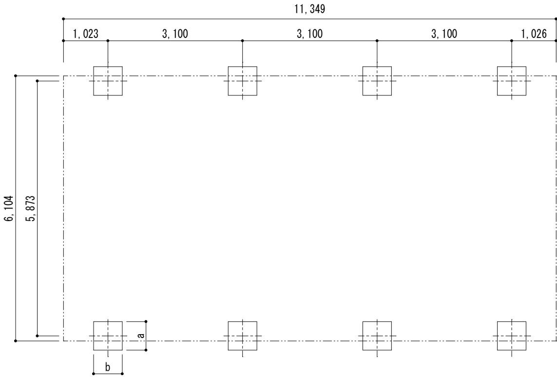
■基礎配置図
